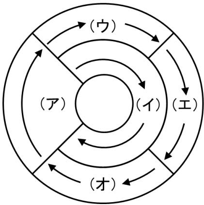
図1．細胞周期
