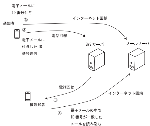
図4 SMSサーバーとIMAPサーバーの双方を利用する安価な構成
