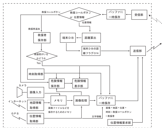
図5 通知者側の詳細な構成例を示すブロック図
